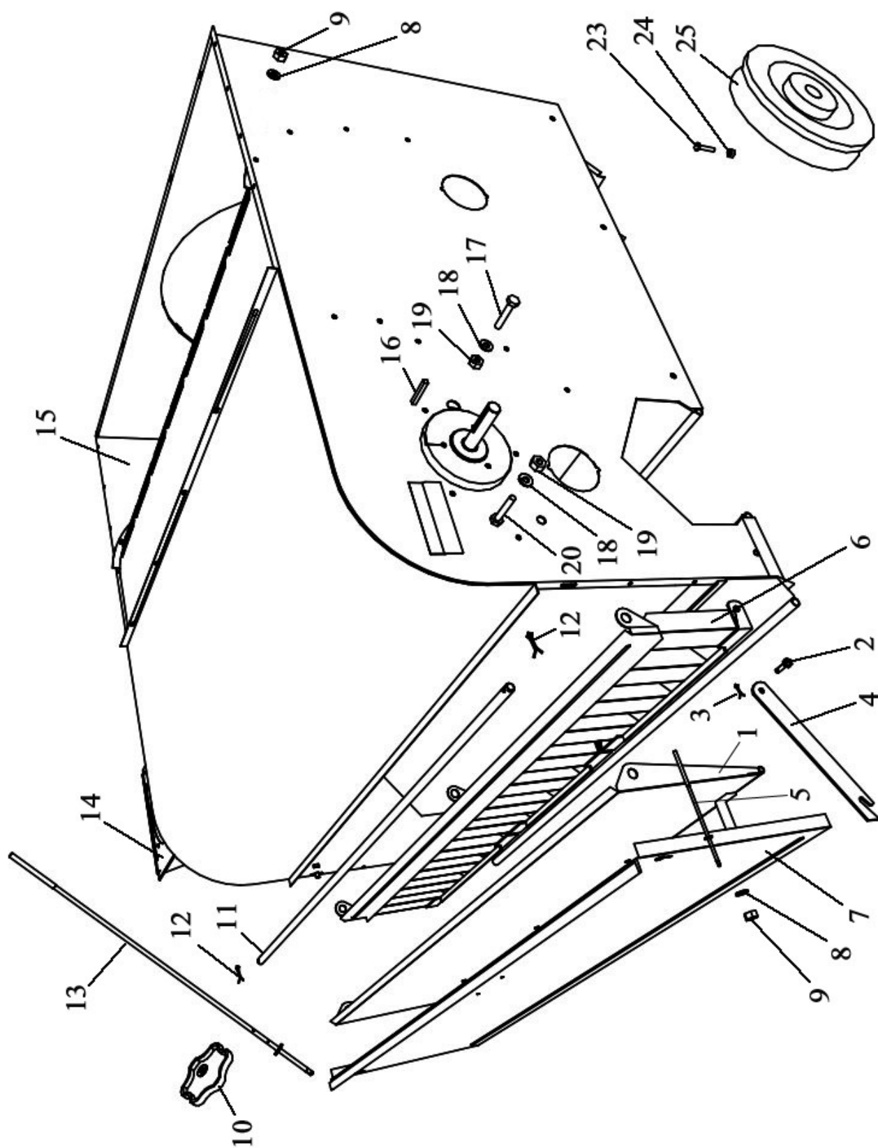
Рис. 3 КАМЕРА ПРИЕМНАЯ
