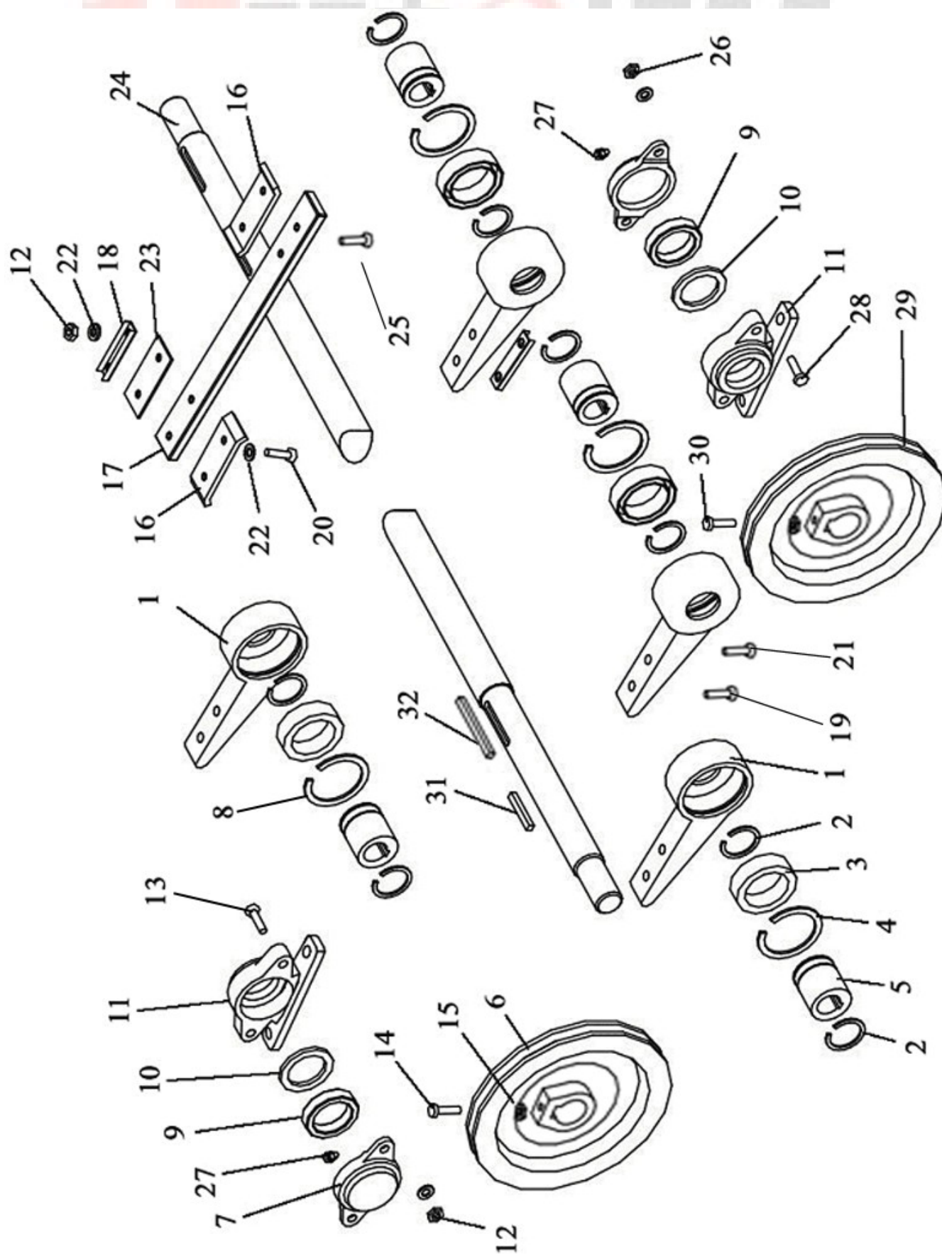
Рис. 8 ПРИВОД ЭКСЦЕНТРИКОВЫЙ
